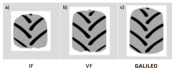
Gemeten voetafdrukken van banden met de verhoudingen 600/65R28CW (a) commerciële IF-band (b) commerciële VF-band (c) TrakWheel
