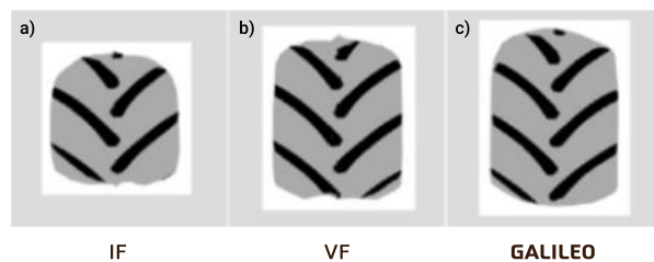
Gemessene Aufstandsflächen von Reifen mit 600/65R28 Proportionen (a) Handelsreifen IF (b) Handelsreifen VF (c) TrakWheel.
