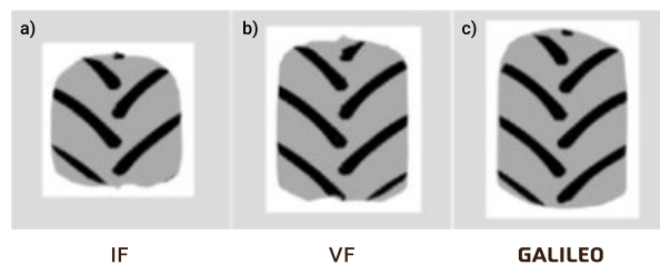
Huellas medidas de los neumáticos con proporciones 600/65R28CW (a) neumático comercial IF (b) neumático comercial VF (c) TrakWheel.
