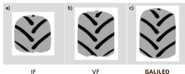
Empreintes de pneus mesurées avec (a) pneu industriel IF, (b) pneu industriel VF, (c) TrakWheel de dimensions 600/65R28CW
