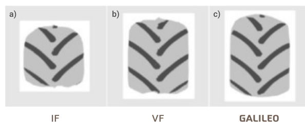
Pegadas de pneus medidas com proporções 600/65R28CW (a) pneu comercial IF (b) pneu comercial VF (c) TrakWheel
